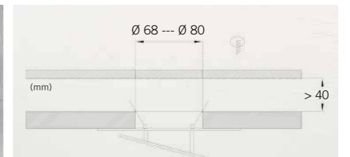
Montageskizze für Einbauleuchte installation draft for built-in light
